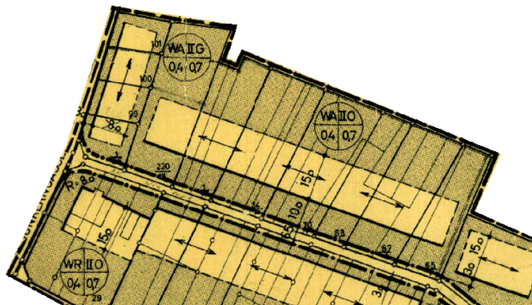
Ausschnitt aus dem Bebauungsplan
